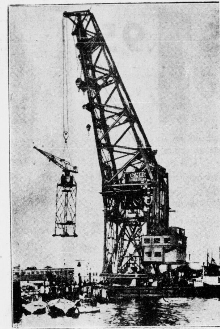
On voit ici une grue flottante de 110 tonnes, à Tokio, Japon, transportant un autre grue, plus petite, mais complète, dans un autre endroit des chantiers maritimes.
